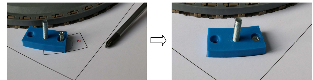
Figuur 6: Montageblokje monteren op sjabloon. Zet de schroef alleen in het rood gemarkeerde gat!
